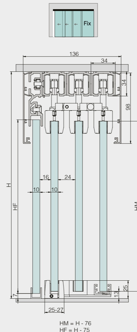
Trascinamento meccanico 3 ante con vetro fisso a soffitto Modelo telescópico mecánico para 3 hojas con vidrio fijo a techo
