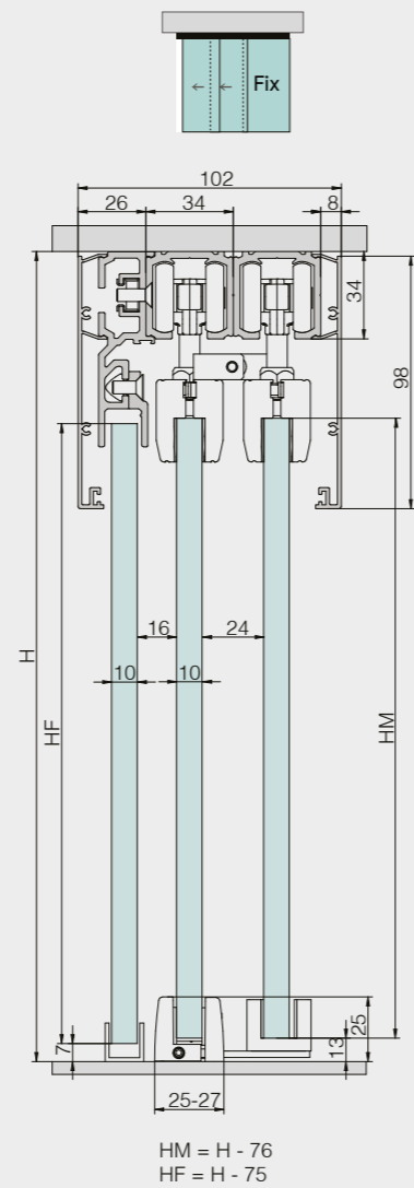
Trascinamento meccanico 2 ante con vetro fisso a soffitto Modelo telescópico mecánico para 2 hojas con vidrio fijo a techo
