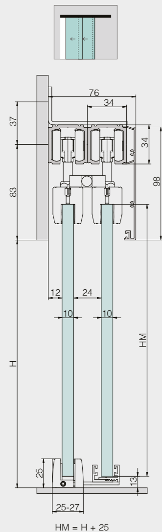
Trascinamento meccanico 2 ante fissaggio a parete Modelo telescópico mecánico para 2 hojas a pared
