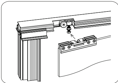
Aggancio anta al control telaio
