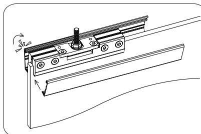
Inserimento a scatto dei carter
