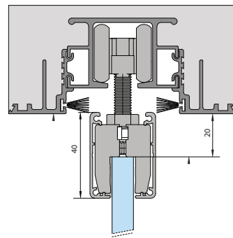
PINZA EASY IN CONTROTELAIO FILO MURO
