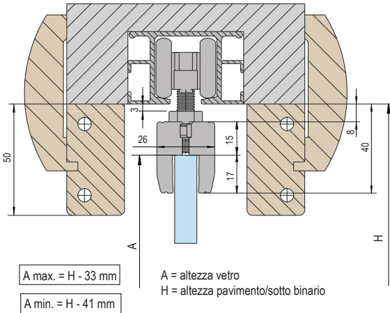
PINZA EASY IN CONTROTELAIO CLASSICO
