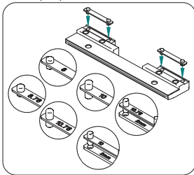
Aggancio anta al control telaio
