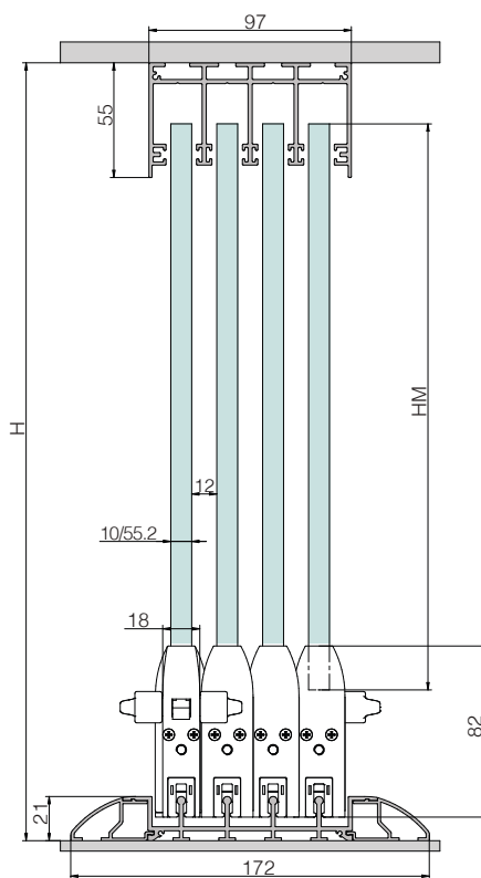
Apertura contrapposta L Max. 10.400 mm
