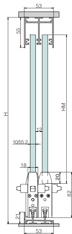
Apertura contrapposta L Max 5.200 mm
