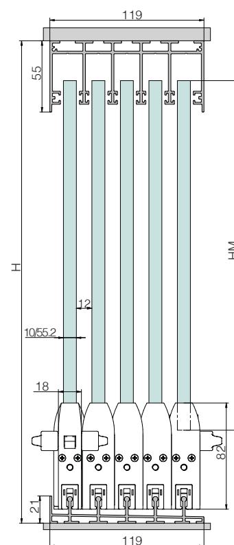
HM = H - 104 In appoggio
