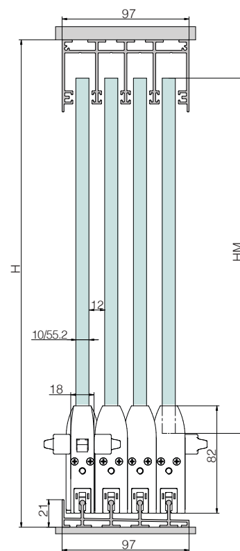
Apertura semplice L Max 5.200 mm
