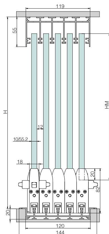
HM = H - 84 Incassata
