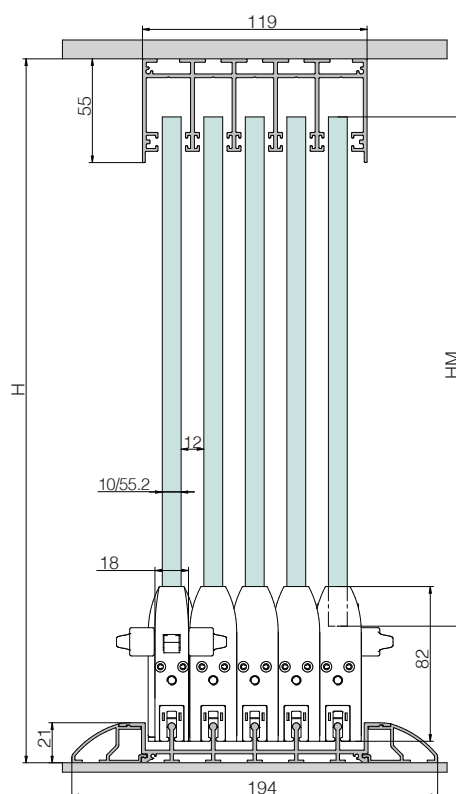
HM = H - 104 A becco d'oca
