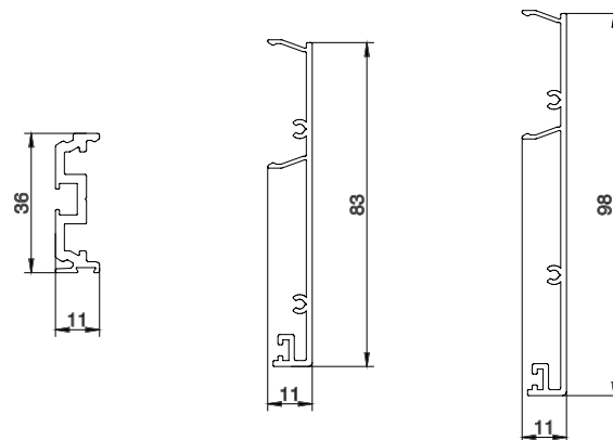
profilo distanziatore
