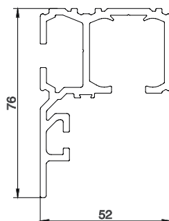
profilo scorrimento con vetro fisso
