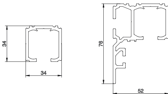
profilo scorrimento anta singola
