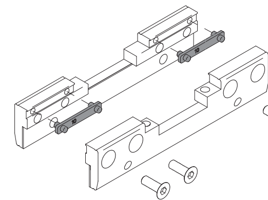
VETRO 12 MM
