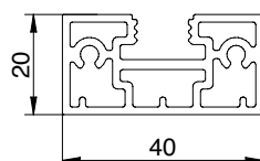
profilo laterale anta
