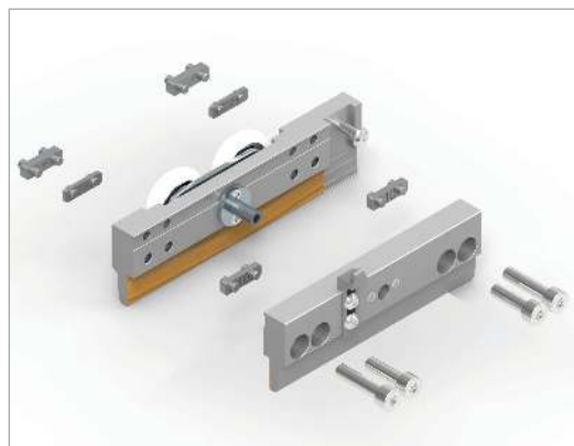
PINZA
